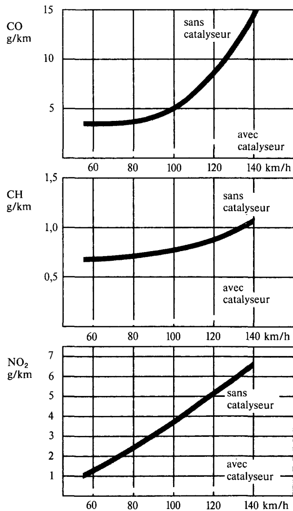
Rejets toxiques provenant d'une voiture de catégorie moyenne, avec et sans catalyseur
